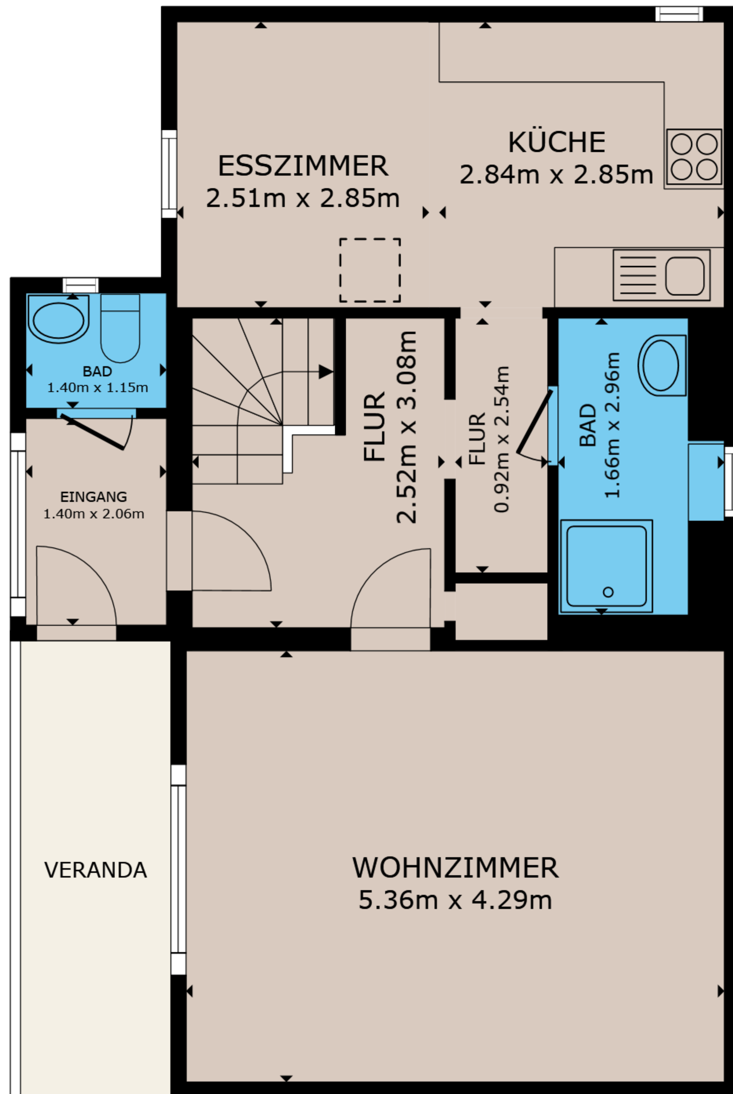
STOCKWERK 1
